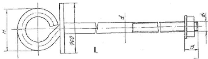
Стяжка винтовая РС
